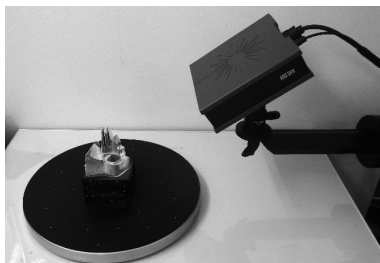
ATOSを使用している計測の様子
