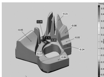
測定結果の表示。3DCADデータをもとに現物との比較をした様子
